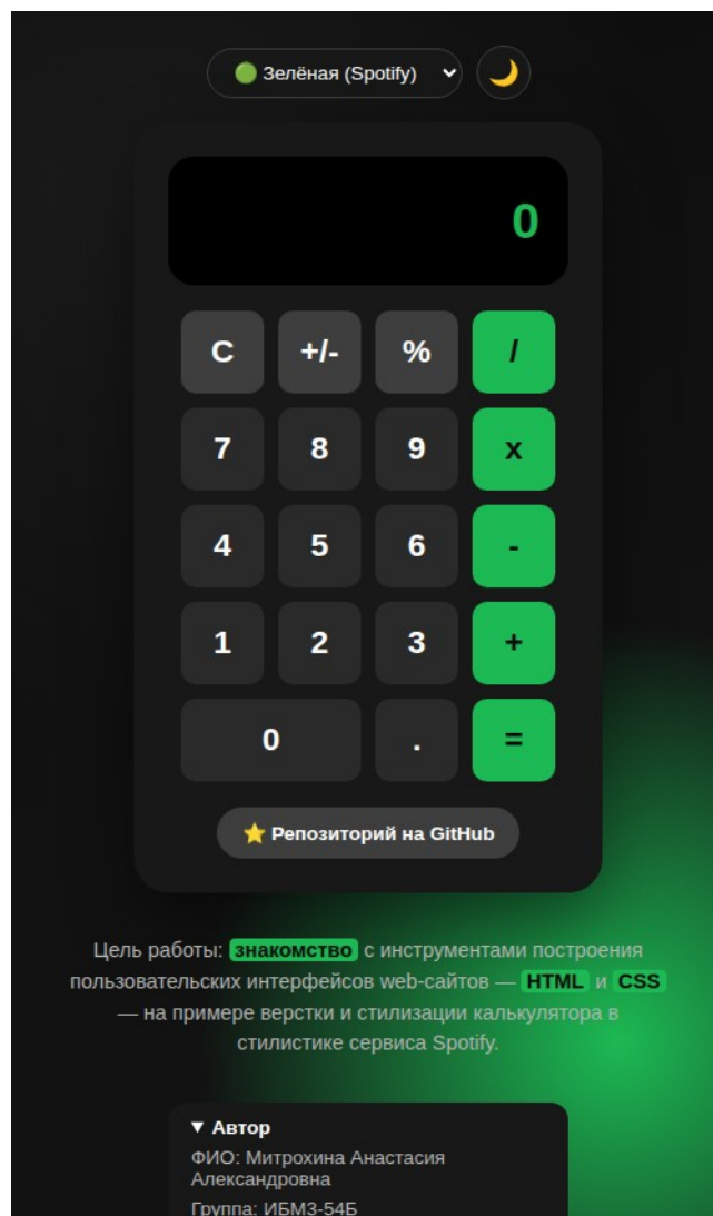
Рис. 3 — Раскрытый блок «Автор» (сворачивающиеся подробности, п.18) и подсветка ключевых слов в цели работы (п.19)
